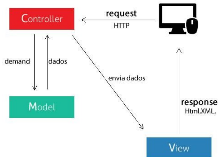
Figura 1. Modelo de arquitetura MVC Fonte: https://tableless.com.br/mvc-afinal-e-o-que/ 4.1.1. Tipos de Teste no framework Laravel
