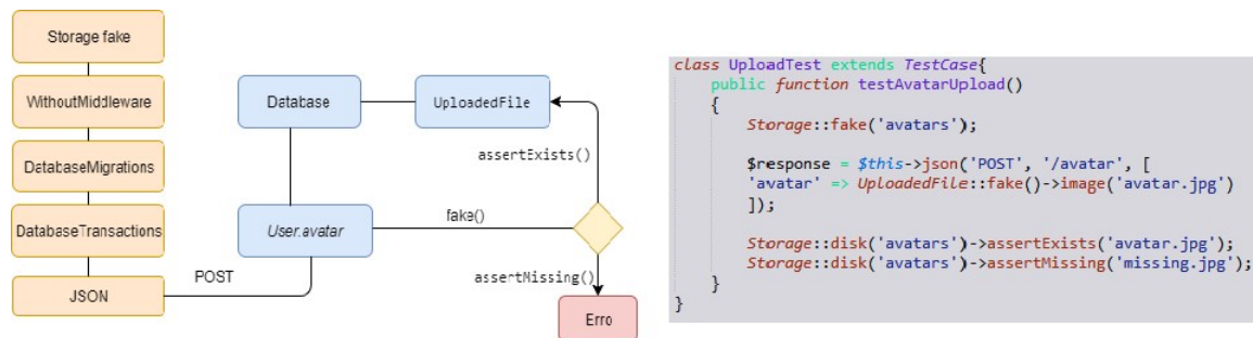
Figura 6. Teste de upload (simulação) (Fonte: dos autores, 2018)
