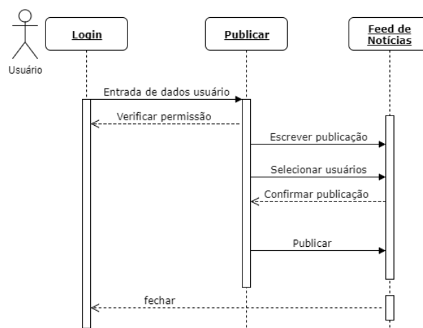
Figura 9. Diagrama de sequência - etapa de especificação de teste manual (Fonte: dos autores, 2018)
