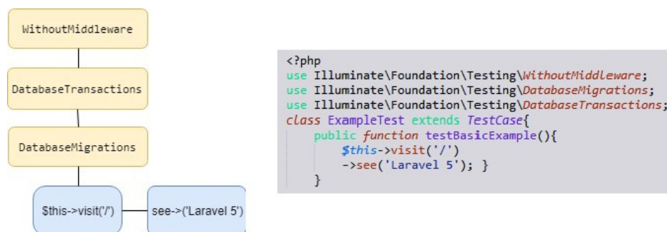
Figura 2. Teste de acesso com uma resposta esperada (Fonte: dos autores, 2018)
