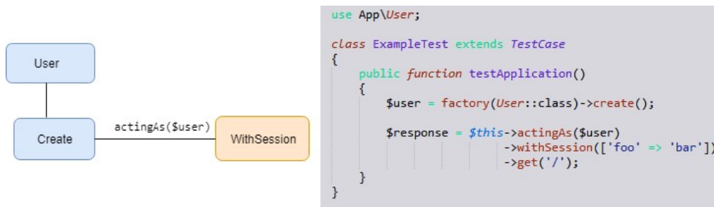
Figura 3. Teste de autenticação de usuário (Fonte: dos autores, 2018)
