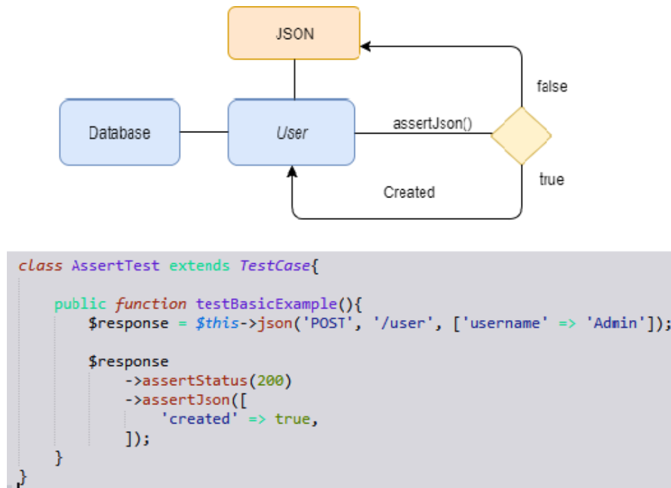
Figura 5. Diagrama de atividades de teste de APIs JSON - Saídas esperadas (Fonte: dos autores, 2018)
