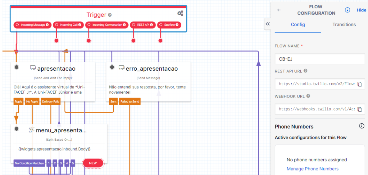
Figura 5 – Segmento do fluxo Twilio Studio
