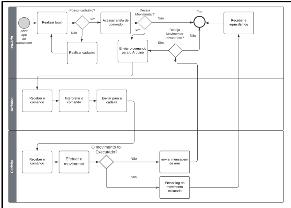
Figura 02 - BPMN
