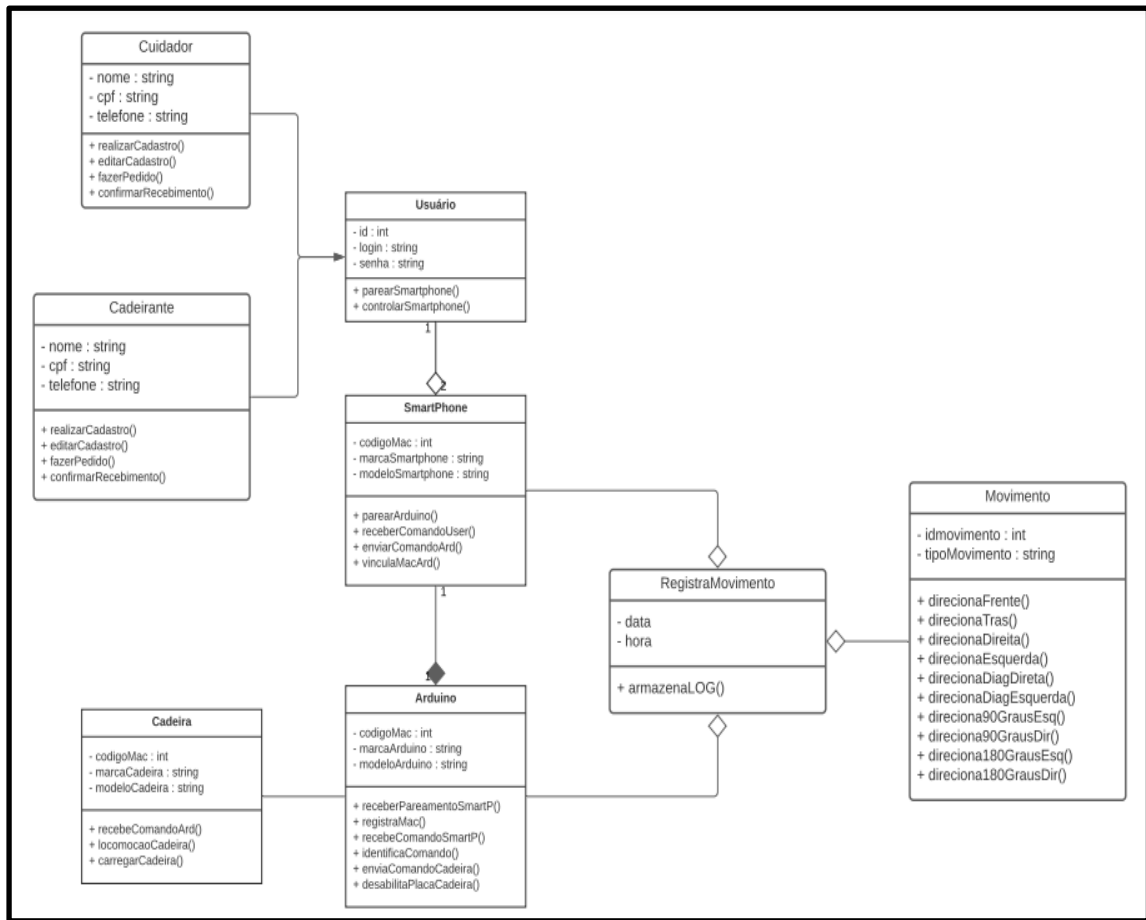
Figura 04 – Diagrama de Classe
